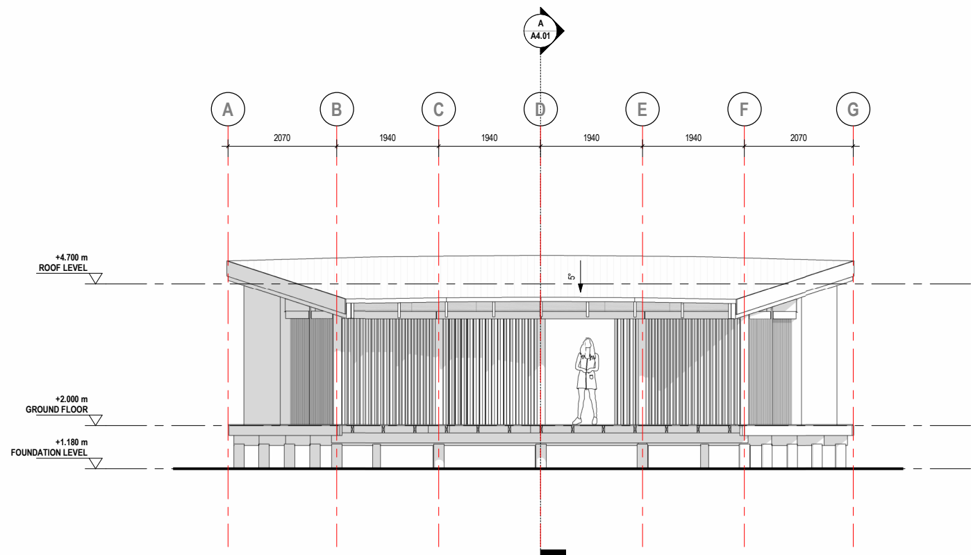
1 FRONT ELEVATION SCALE: 1 : 50
