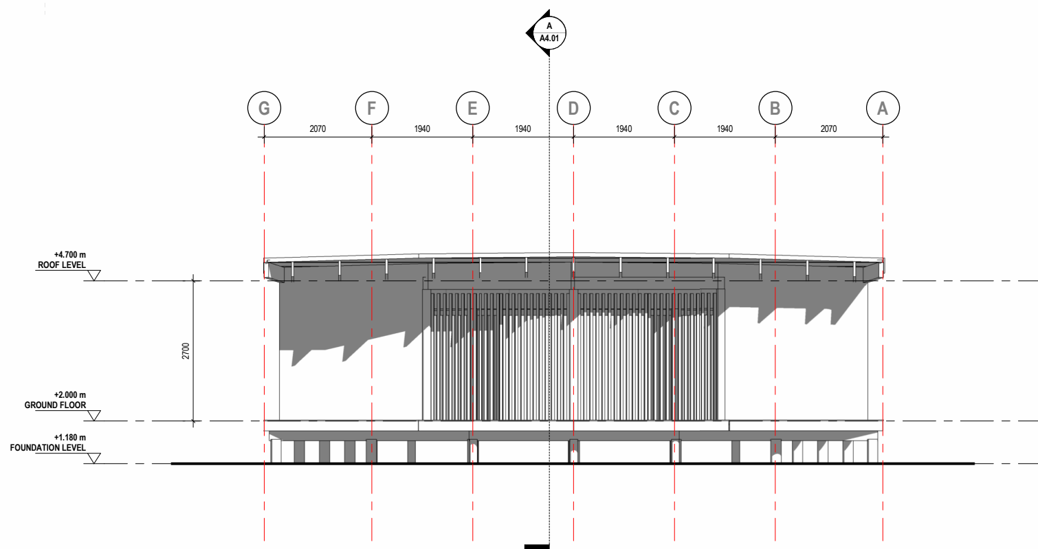
2 REAR ELEVATION SCALE: 1 : 50
