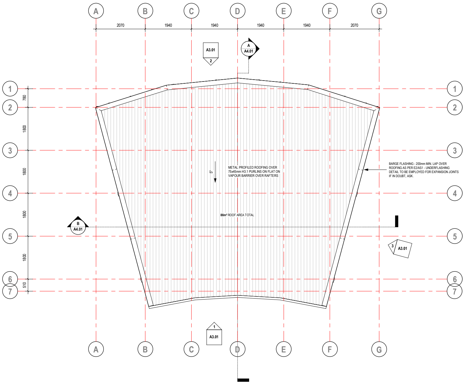
1 ROOF PLAN A3.01 SCALE: 1 : 50
