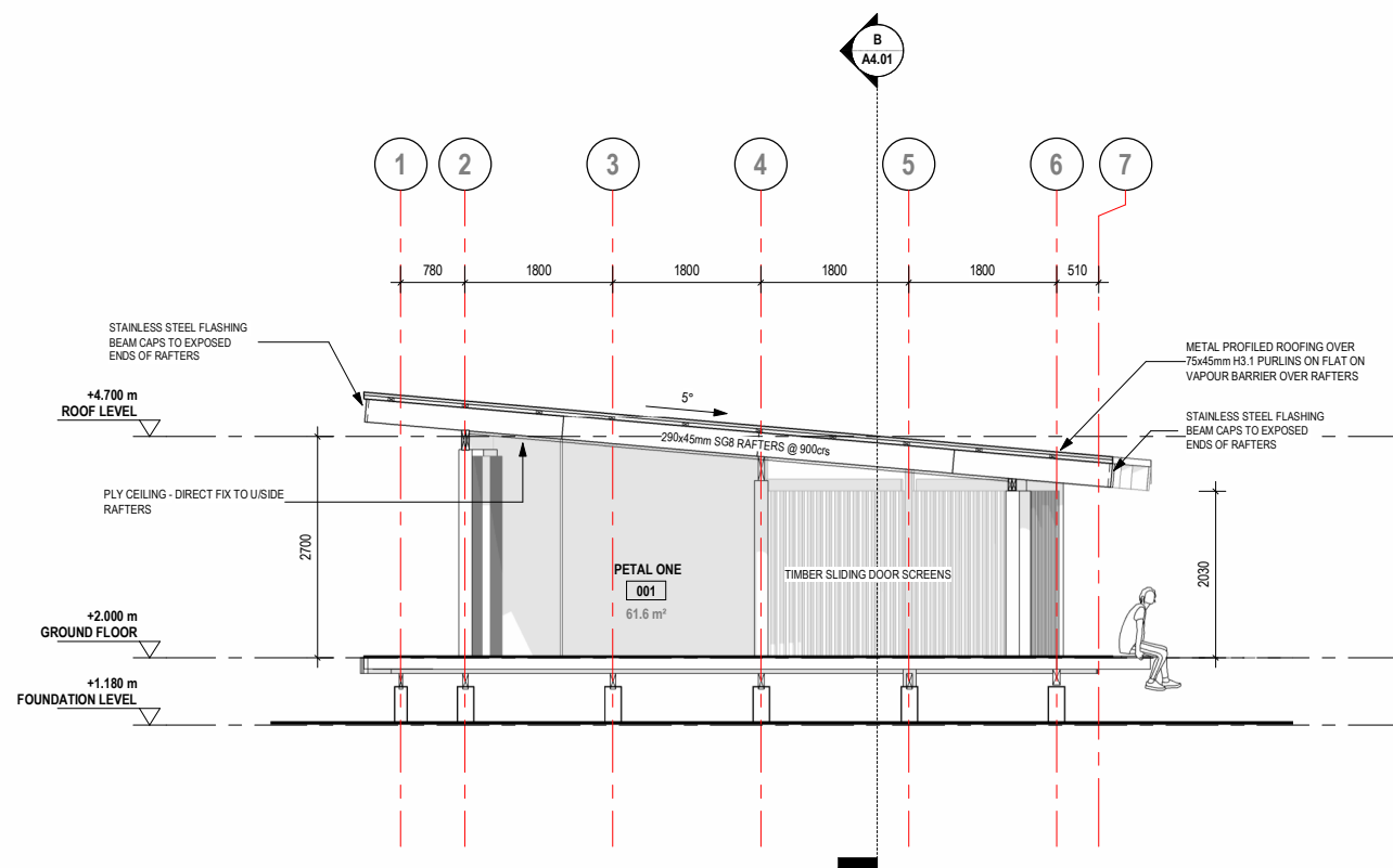
A A2.00 SECTION A-A SCALE: 1 : 50
